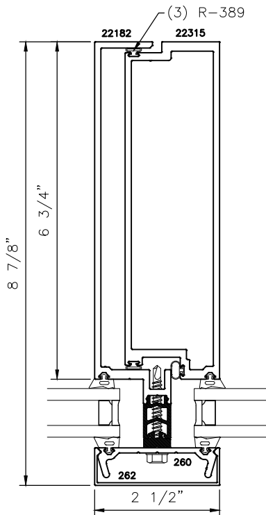
OPT. 5.2
