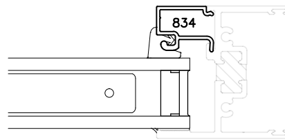
RIGHT JAMB
