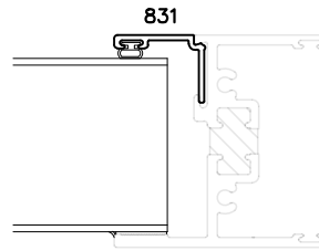
RIGHT JAMB
