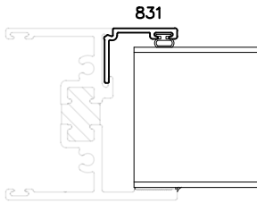
LEFT JAMB
