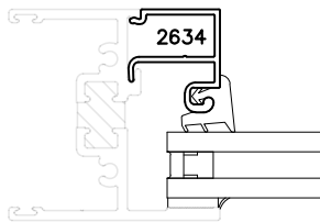
LEFT JAMB
